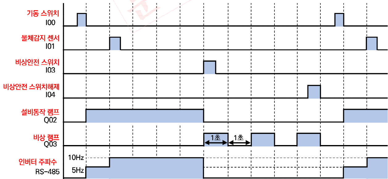
[기동 중 비상안전 스위치 작동]
